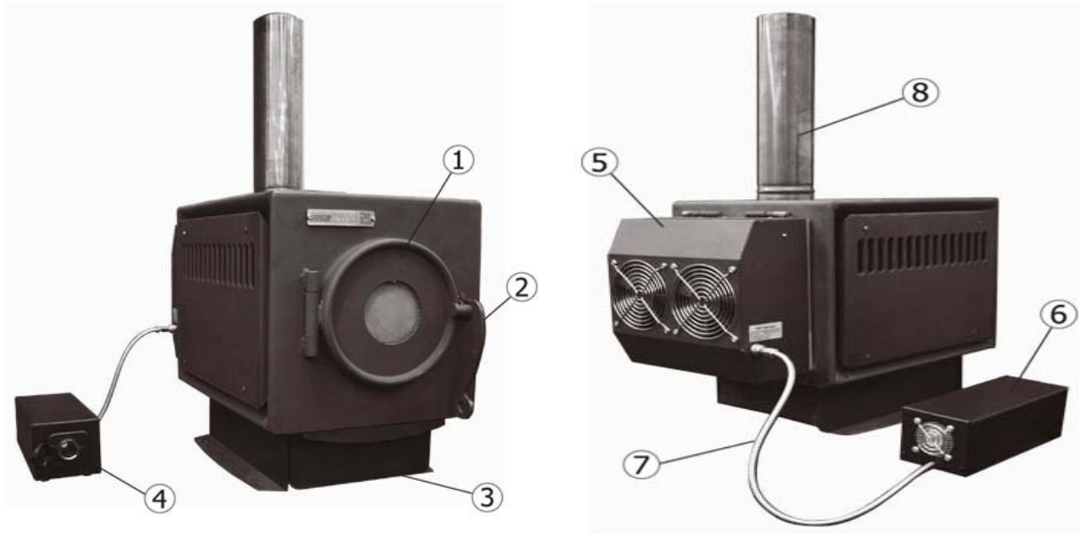
Рис. 1. Внешний вид изделия Энергопечь. 1- дверца топливника, 2- ручка дверцы топливника, 3 – выдвижной зольный ящик, 4 – гнездо для подключения нагрузки; 5 – термоэлектрический генератор, 6 – блок стабилизации напряжения, 7- бронированный кабель, 8 — дымоход.
